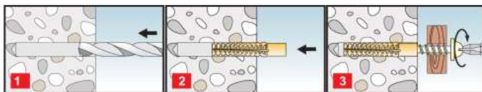
Рис. 2. Установка дюбеля КФСТ.735322.095 и КФСТ.735322.096.
